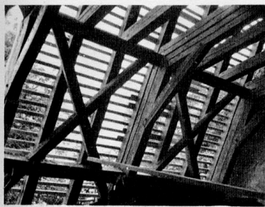
Balkenkonstruktion im Chor.
